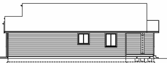
RIGHT ELEVATION
