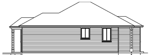
RIGHT ELEVATION
