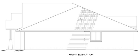
RIGHT ELEVATION
